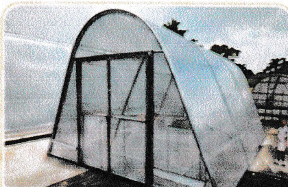
ระบบอบแห้งครัวเรือน ขนาด 4.6 x 6.40 เมตร
