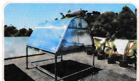
ระบบอบแห้งขนาดเล็ก ขนาด 1.5 x 2.00 เมตร
